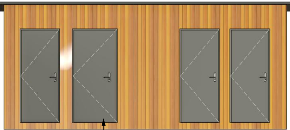
5 Elevation E 1 : 50
